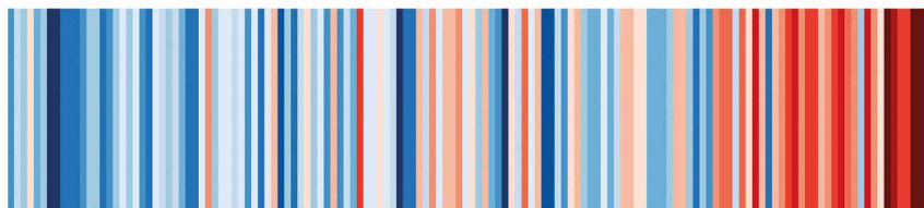
ABBILDUNG 1: WARMING STRIPES
